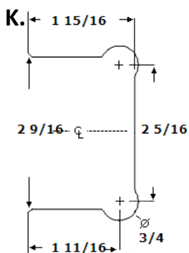
Hinge Cutout 'K' 2.5625"W x 1.9375"D
