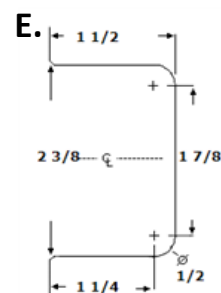
Hinge Cutout 'E' 2.5"W x 1.5"D - Pivot
