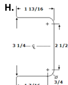
Hinge Cutout 'H' 3.25"W x 1.8125"D - Pivot
