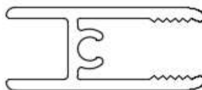
Top/Bottom Door Rail E-GSCH (E-552)
