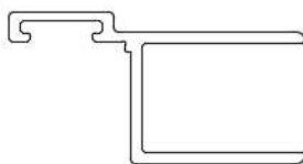
Framed Strike Jamb E-SJF (E-554)
