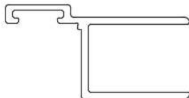
Framed Strike Jamb E-SJF (E-554)
