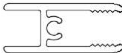
Top/Bottom Door Rail E-GSCH (E-552)
